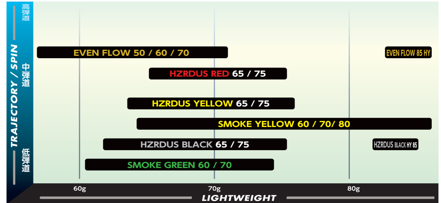
Graphite Shaft Matrix グラファイトシャフト・マトリックス / 重量帯・弾道比較 (カット前重量帯)
